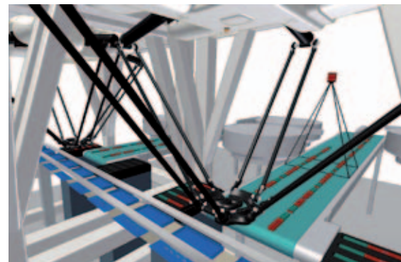
Layout einer Anlage für Lebensmittel (Verpackung in Kartons)
